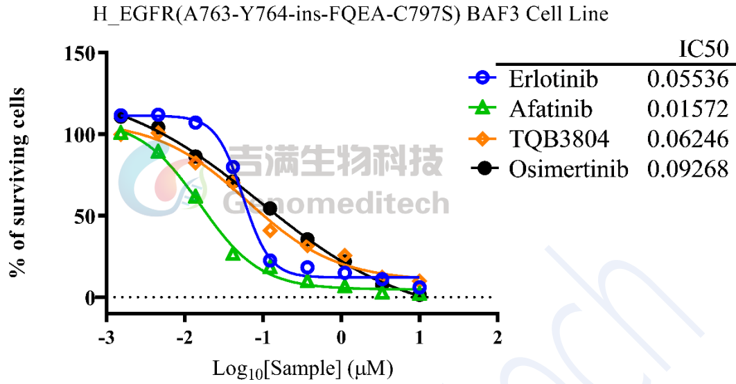
Fig 1. H_EGFR(A763-Y764-ins-FQEA-C797S) BAF3 Cell Line 使用 Erlotinib、Afatinib、TQB3804、Osimertinib 杀伤验证结果。换算方法：活细胞百分比=（加药孔-assay buffer 孔）/（不加药孔-assay buffer 孔）
